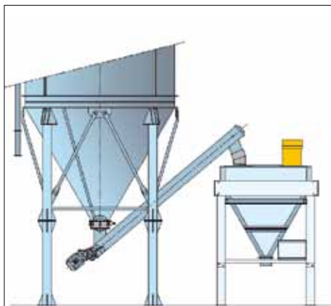
Weigh hopper loaded by screw feeder Behälterwaage durch Dosierschnecke befüllt Trémie alimentée par vis doseuse Dosatore alimentato da codlea estraitrice da silo
