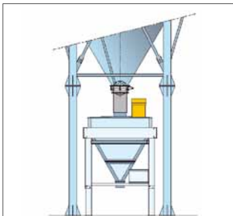
Weigh hopper gravity-fed by silo Behälterwaage unter Silo Trémie alimentée directement par silo Dosatore alimentato da silo
