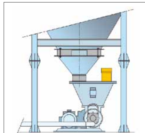
Blow-through rotary valve and pneumatic conveying system Durchblassechleuse und pneumatische Förderung Trémie d'écluse rotative pour transport pneumatique Sfilato rotocella con trasporto pneumatico
